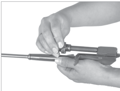
Sl. 10 Odvajanje tela zatvarača od nosača zatvarača
