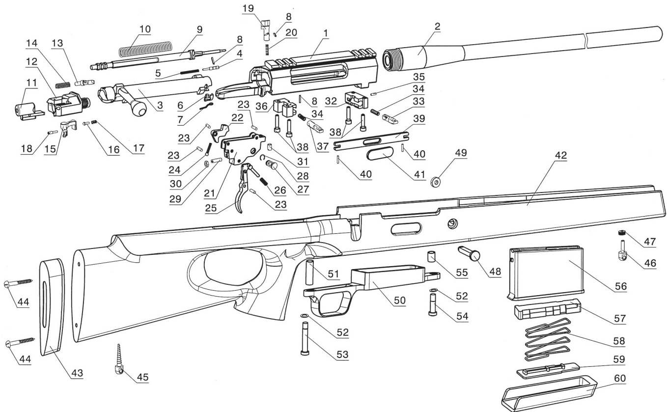
Слика 12 - Ловачки карабин М808 –саставни делови
