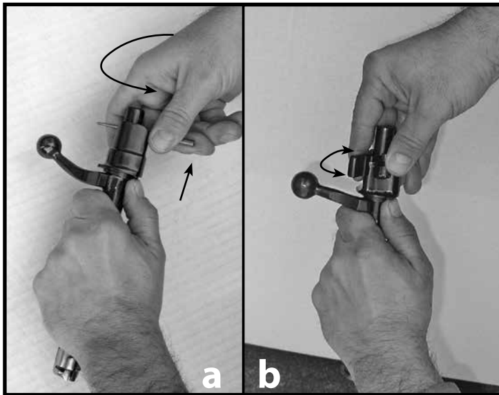
Sl. 16> Odvajanje udarnog mehanizma a) kod modela M70, M70PS, M70PSS i M85; b) kod modela M98
