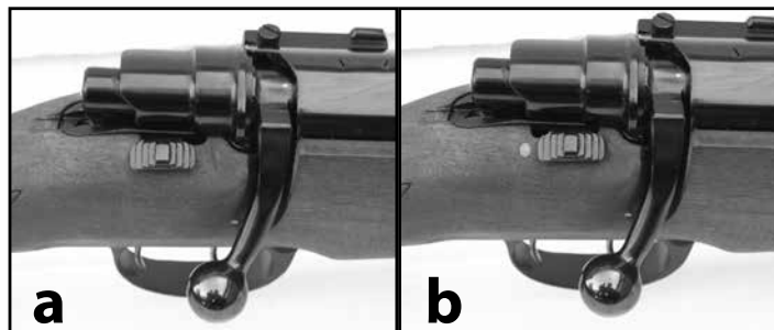
Sl.11> Kočnica karabina kod M70, M70PS, M70PSS i M85 a) položaj kočnice "ukočeno", b) položaj kočnice "otkočeno"
