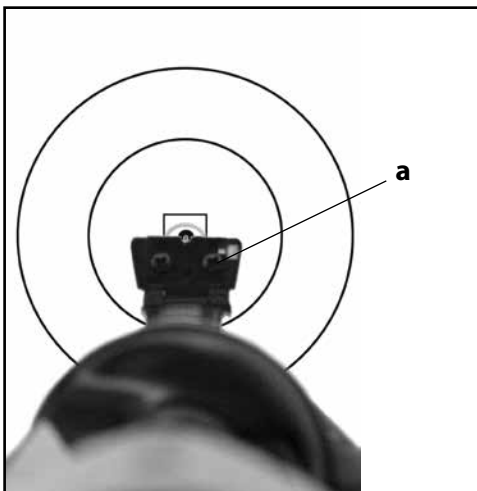
Sl. 19> Postupak nišanjenja a) vijak za podešavanje zadnjeg nišana
