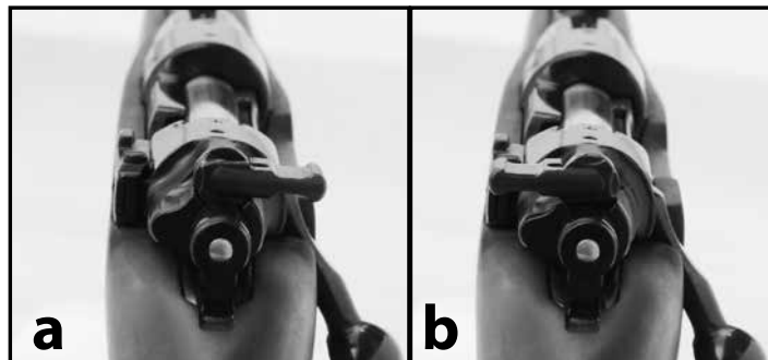
Sl.12> Kočnica karabina kod M98 a) položaj kočnice "ukočeno", b) položaj kočnice "otkočeno"
