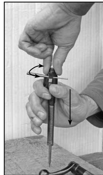
Sl. 17> Rasklapanje udarnog mehanizma
